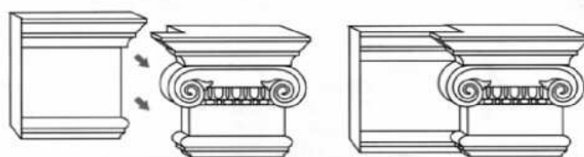
Схема монтажа
